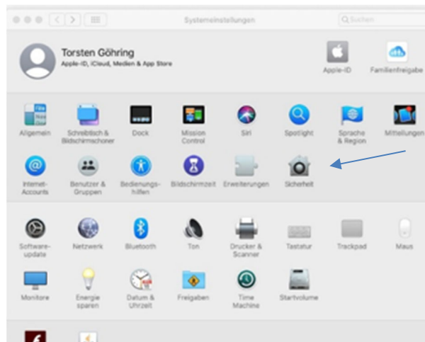
Abbildung 3 Systemeinstellungen
