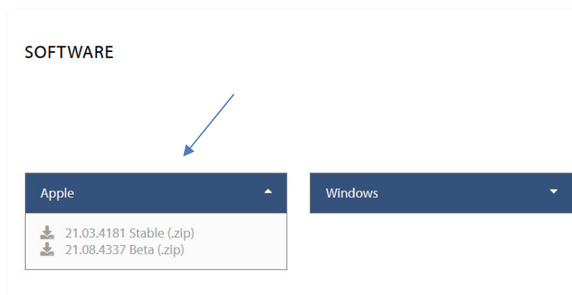
Abbildung 1 Webseite ARTECO
